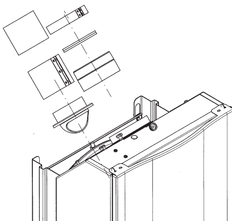
Пример расположения воздуховода (трубы подачи воздуха) слева
